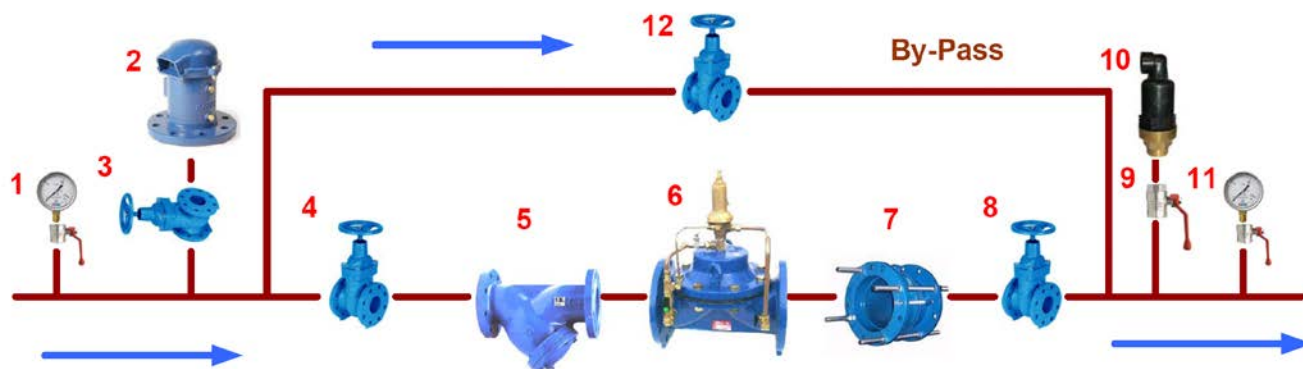
Рис. 8. Рекомендованная схема включения регулятора.
