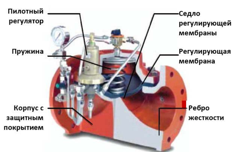
Рис.1. Состав клапана.
